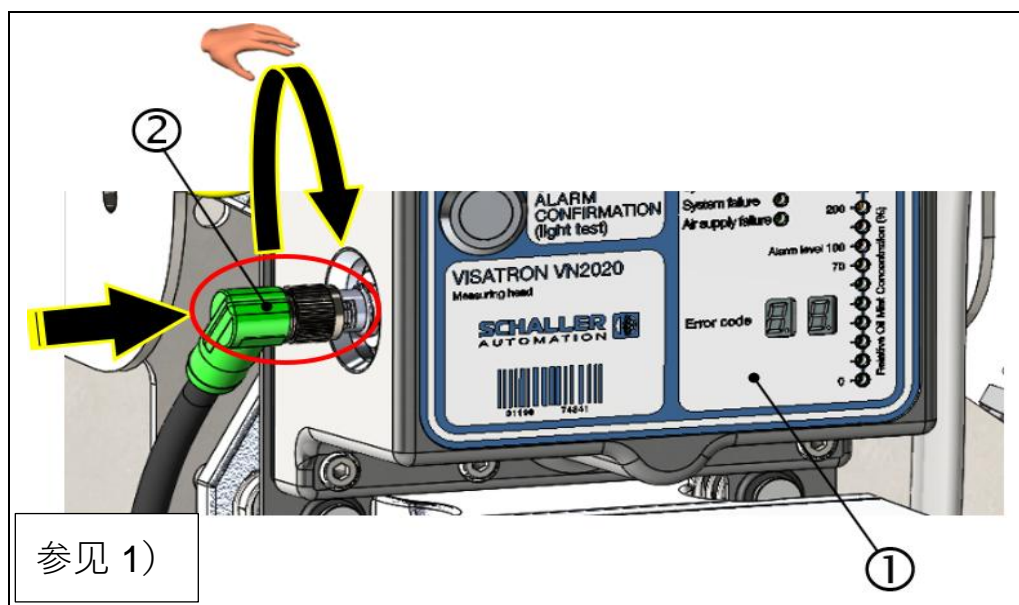
圖: 88: 拆卸接线盒, VN2020 (装配步骤 1 - 8)
