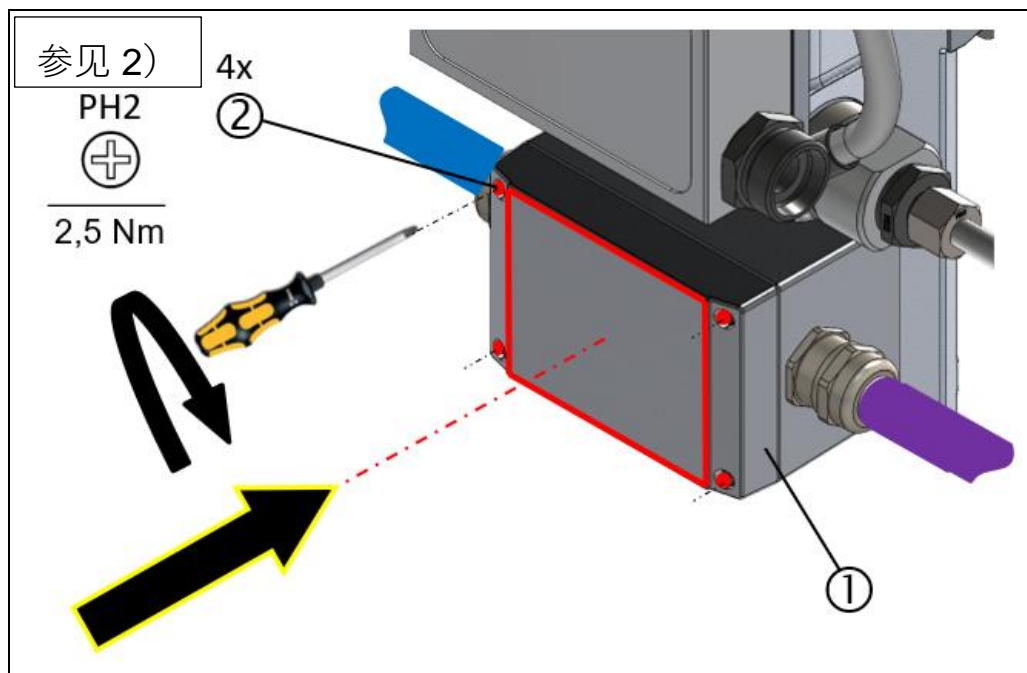
圖: 88: 拆卸接线盒, VN2020 (装配步骤 1 - 8)
