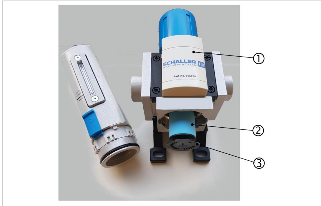
圖: 77: 更換空氣濾清器濾芯, 壓力控制器單元
