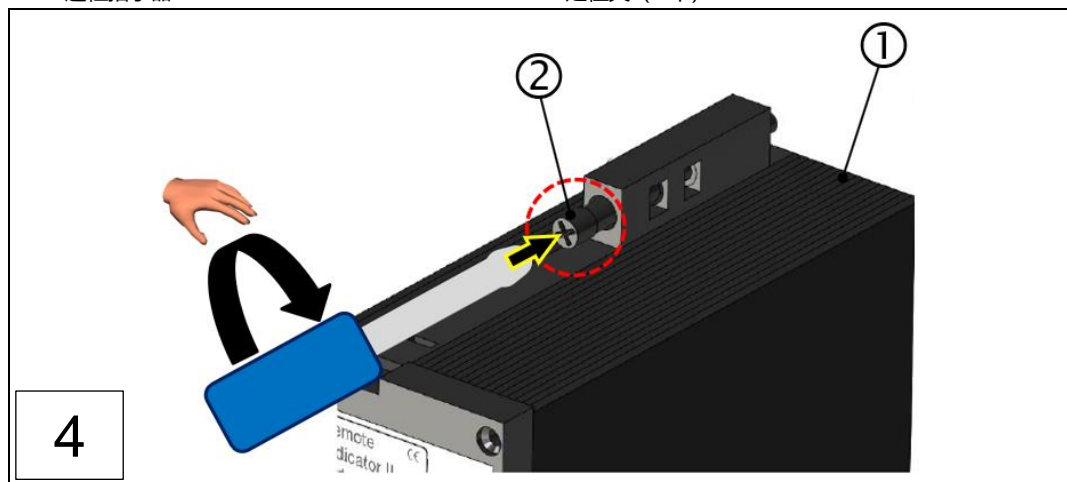
圖: 40: 装配远程指示器 II (装配步骤 1 - 4)
