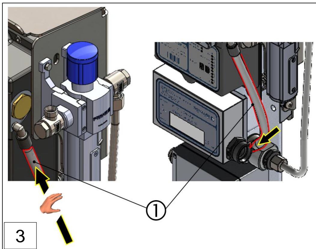
1: 连接软管 (新)
