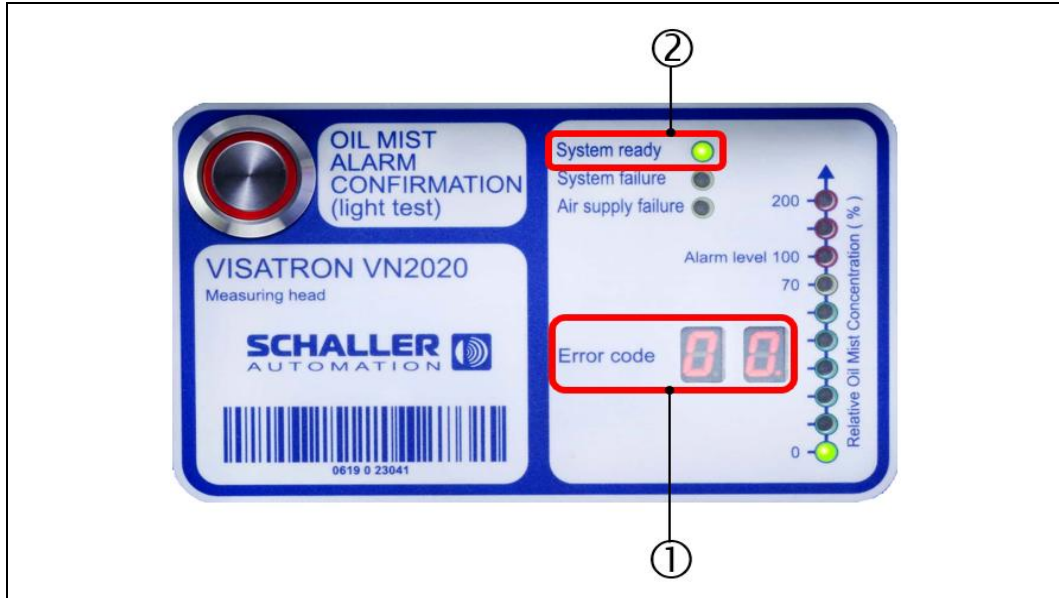
图: 93: 测量附件 VN200: “系统故障或设备故障”状态指示器
