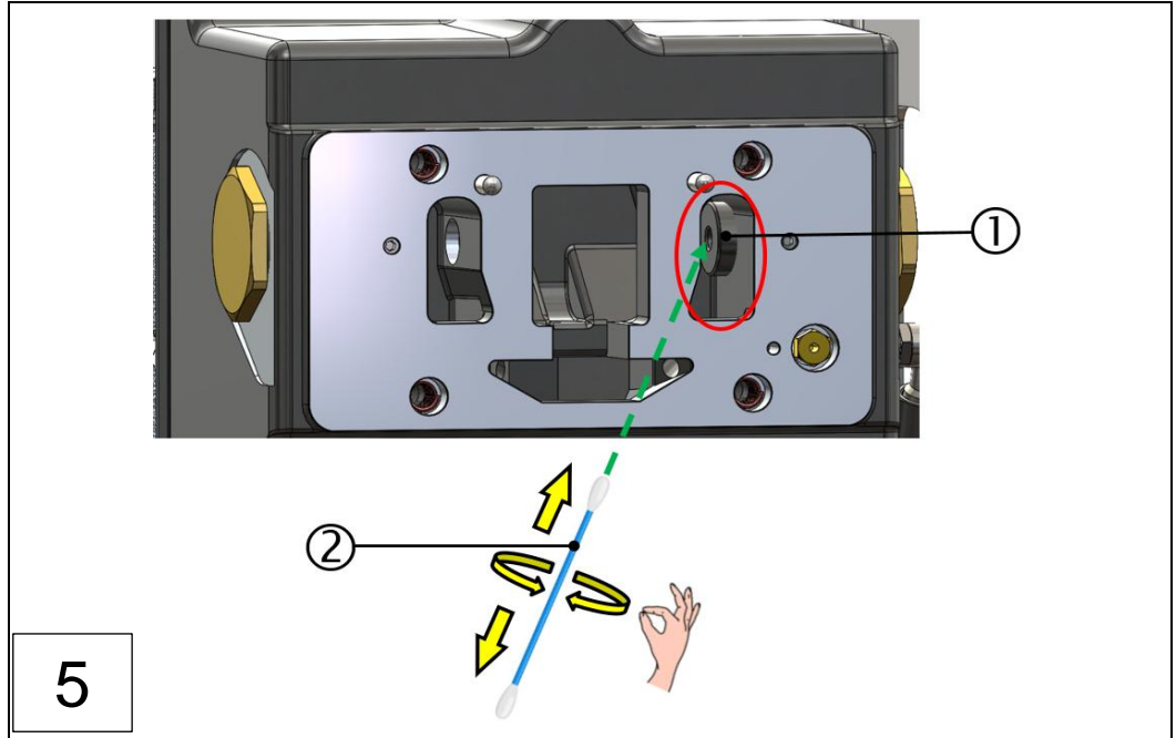
1: 二极管玻璃, 右侧
