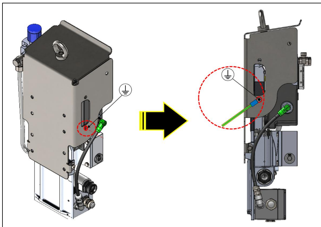
圖: 54： 位置和安装，接地连接、VN200 防护罩
