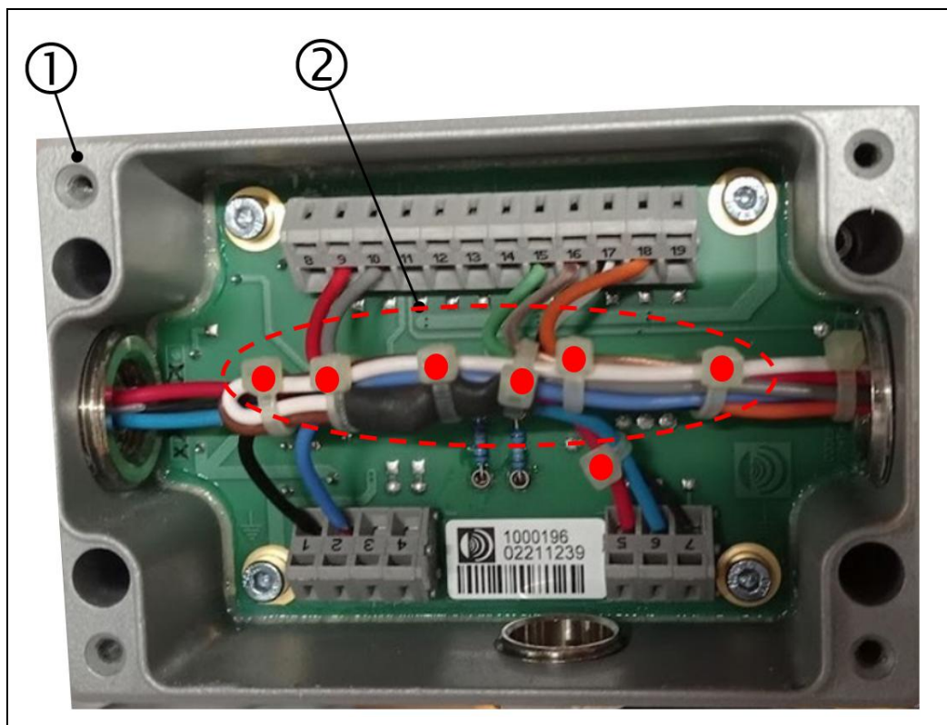
圖: 48: 推荐的电气安装, VN200 接线盒
