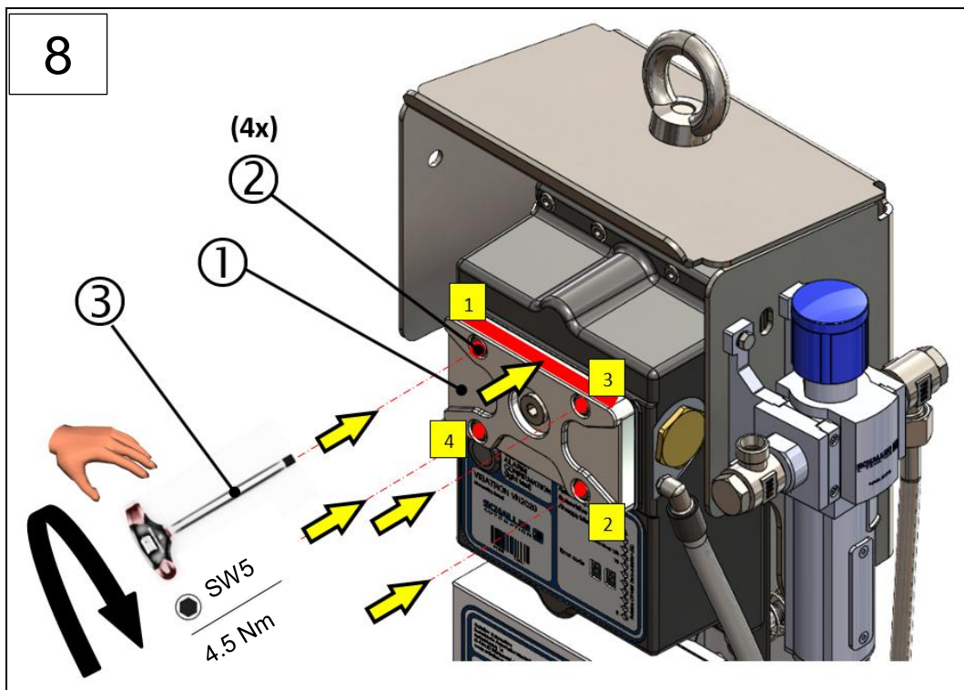
圖: 75: 清洁光路, VN200 (步骤 1 - 8)
