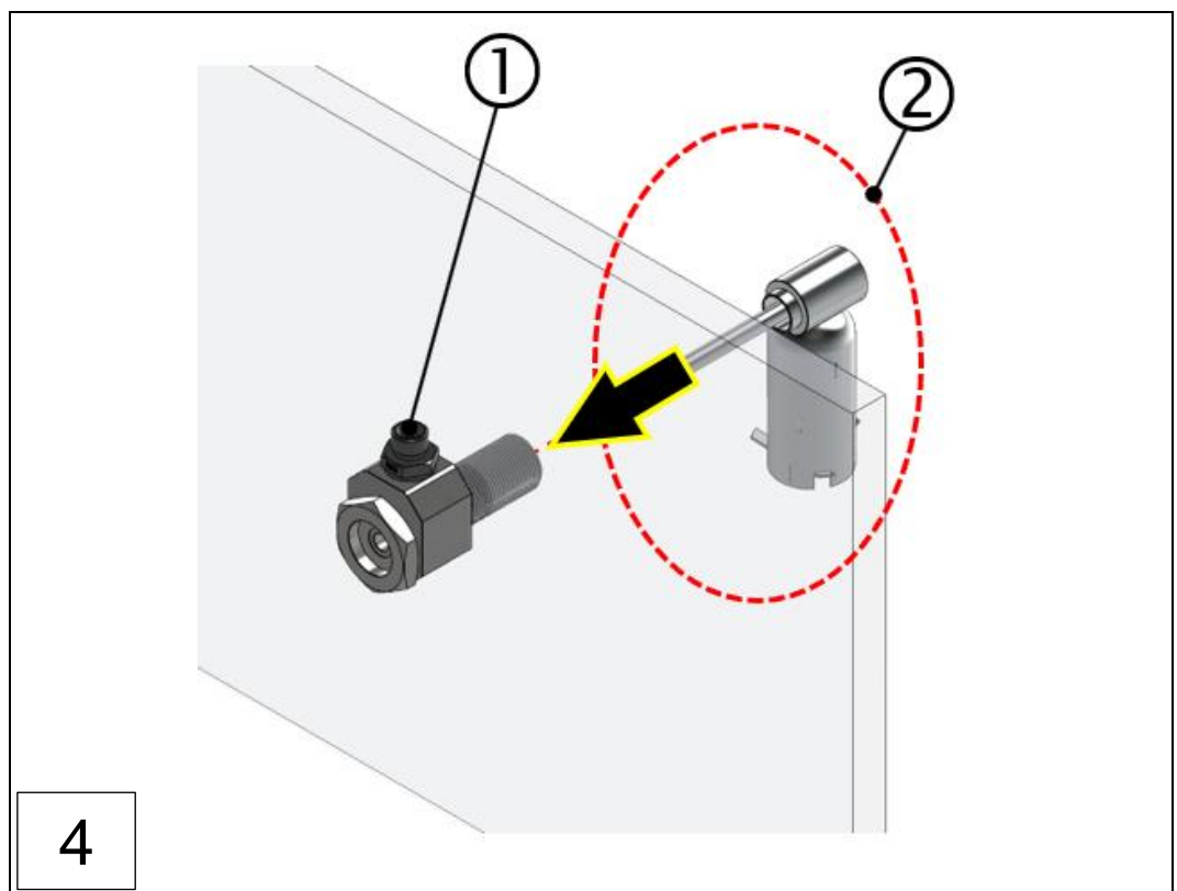
1: 螺栓连接体
