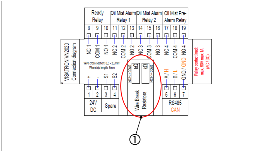
图: 44: VN2020 接线盒: 断路电阻的配置
