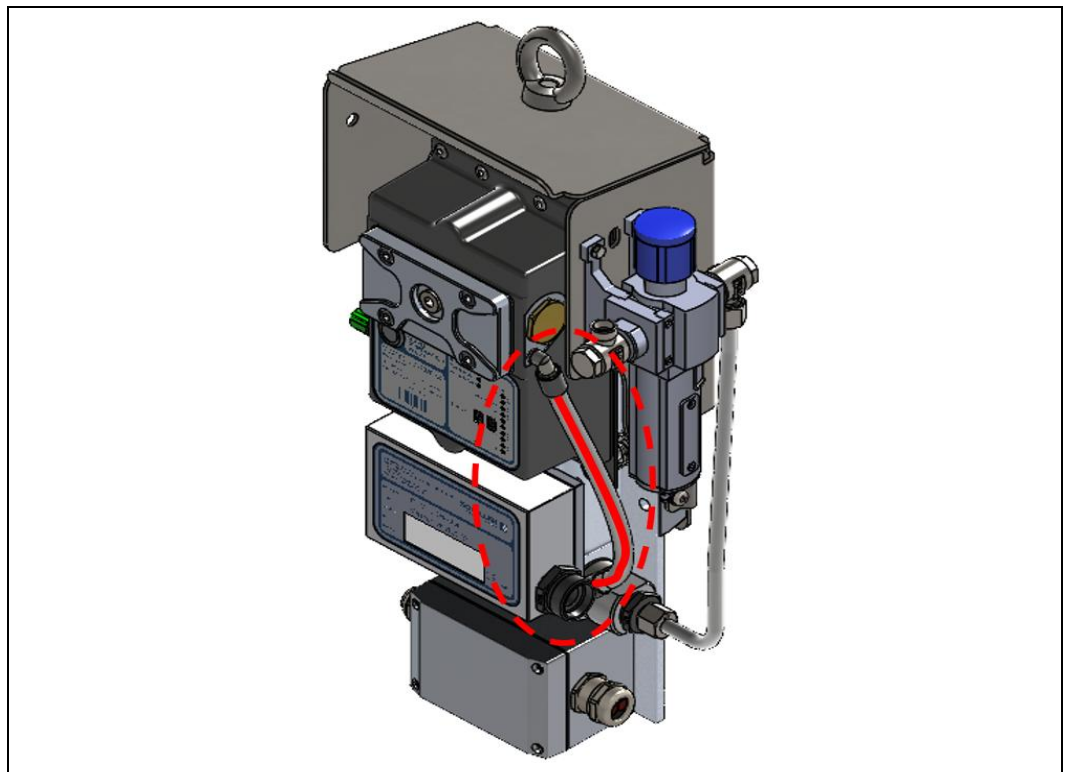
圖: 91: 连接软管, VN2020 油雾探测器
