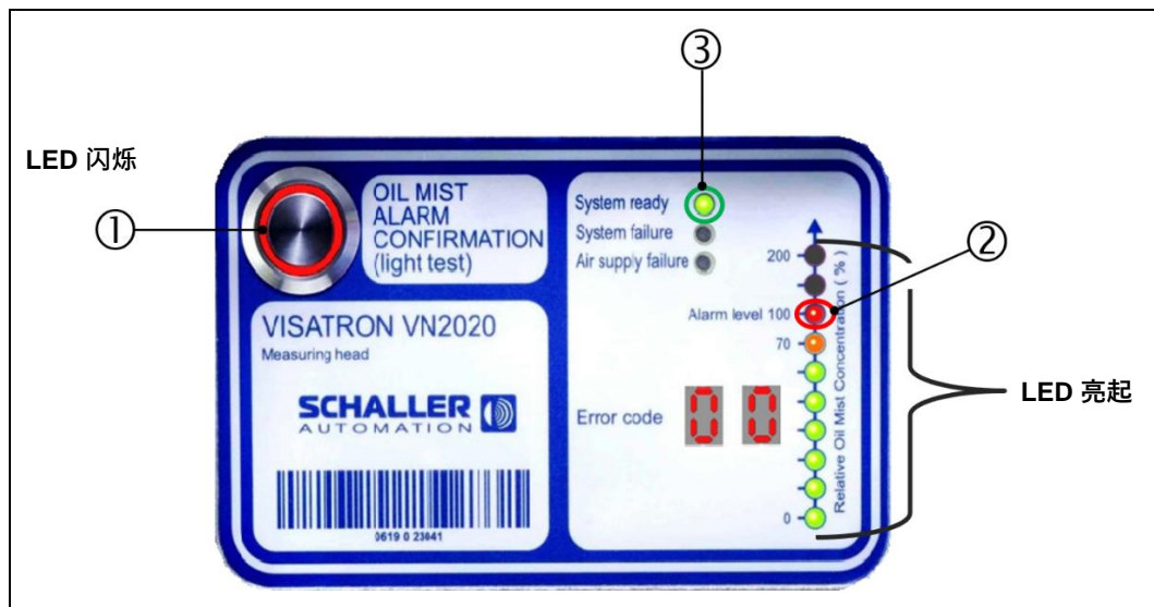
圖: 72： 測量附件 VN2020：100% OMC 時的“报警”状态指示器
