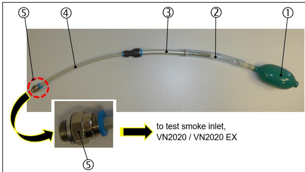
图：79： 烟雾测试盒 (151780) 中的烟管及手摇泵（已装配）
