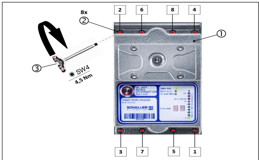
图: 68： VN2020 测量附件的装配
