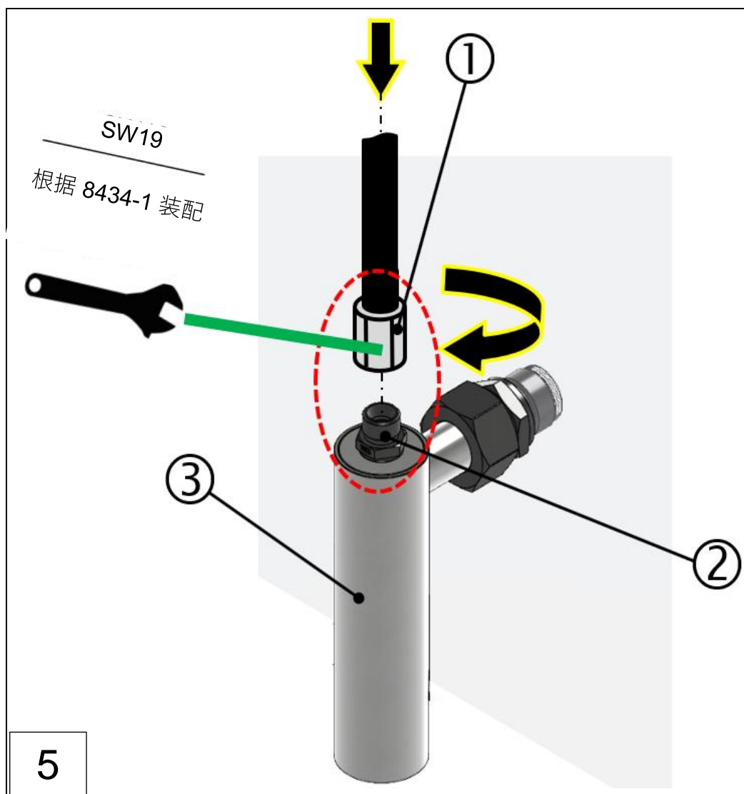
图: 33: 虹吸瓶组件的装配及投入使用 (装配步骤 1 - 5)
