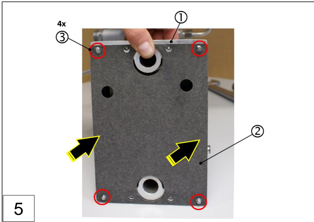
1: 测量附件 (新), VN2020 3: 凸缘螺栓
