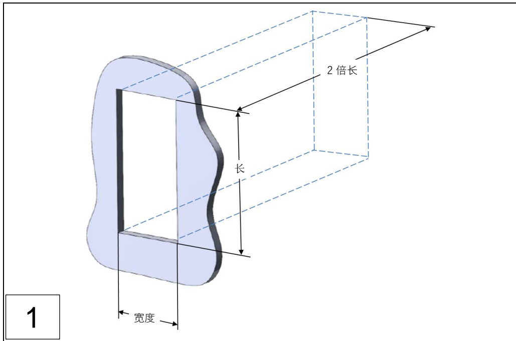
圖: 39: 安装空间尺寸, 远程指示器 II
