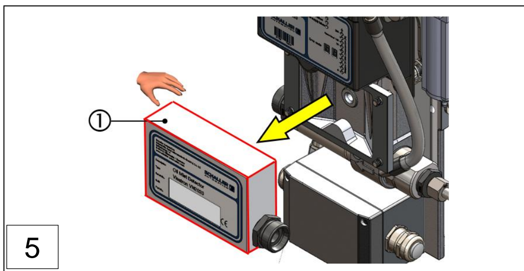
1: 连接箱, VN200
