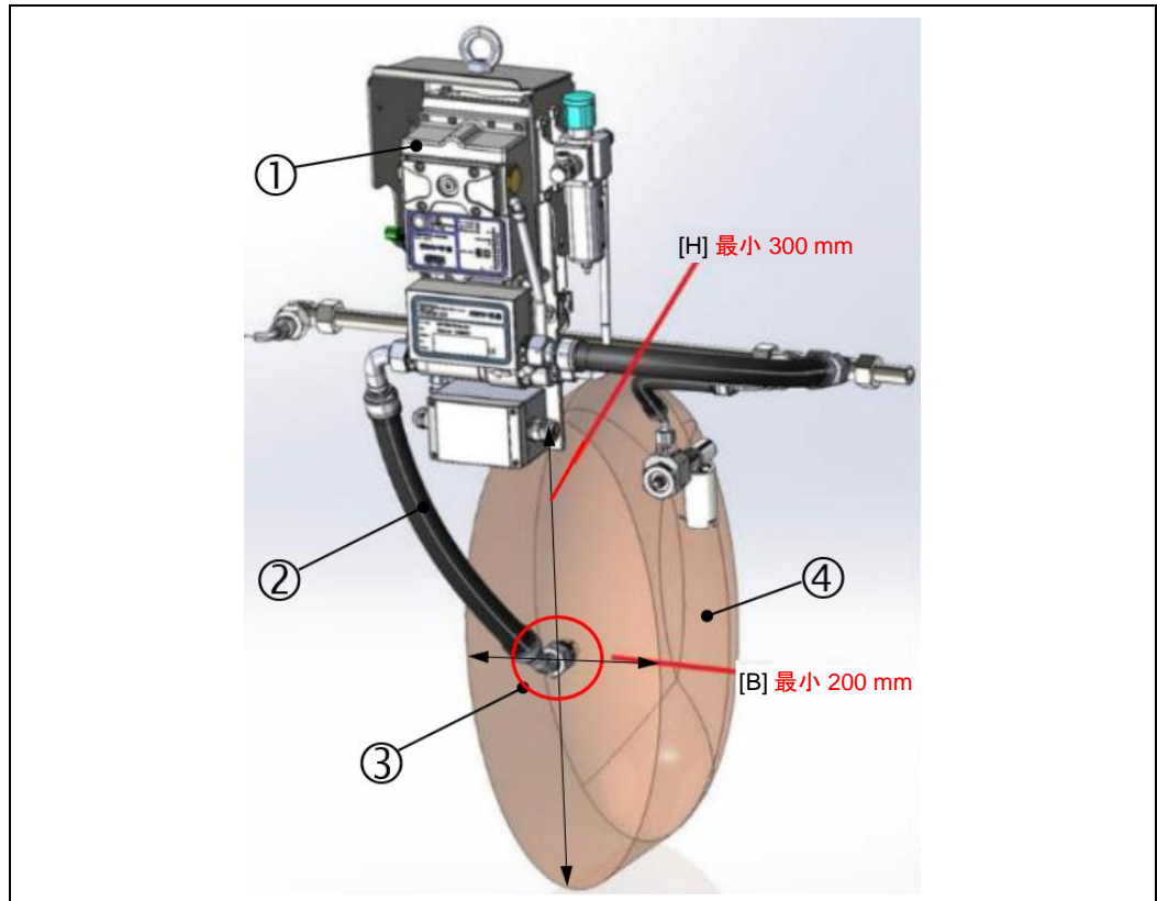
图: 35: 回输管路的位置, VN2020
