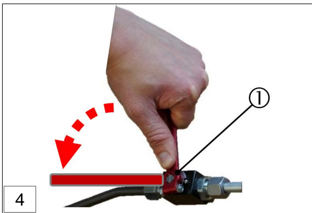
圖: 92: 更換連接軟管, (步驟 1 - 4)
