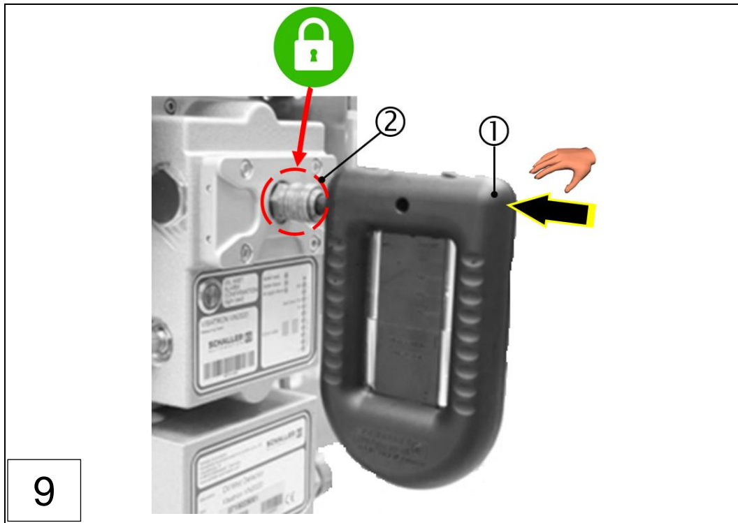
圖: 84 : 更換測量附件, VN2020 (步驟 1 - 9)
