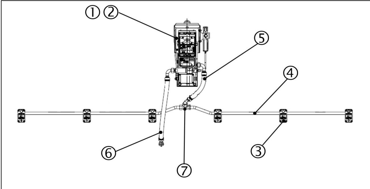
圖: 11: 组件概览, 采用虹吸管组的排水方案, VISATRON® VN200
