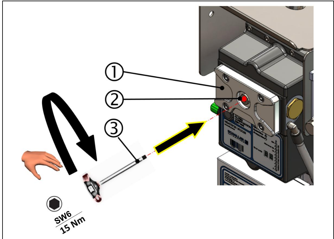
圖: 58 : 將螺旋塞在測量附件上旋入, VN2020 / VN2020 EX
