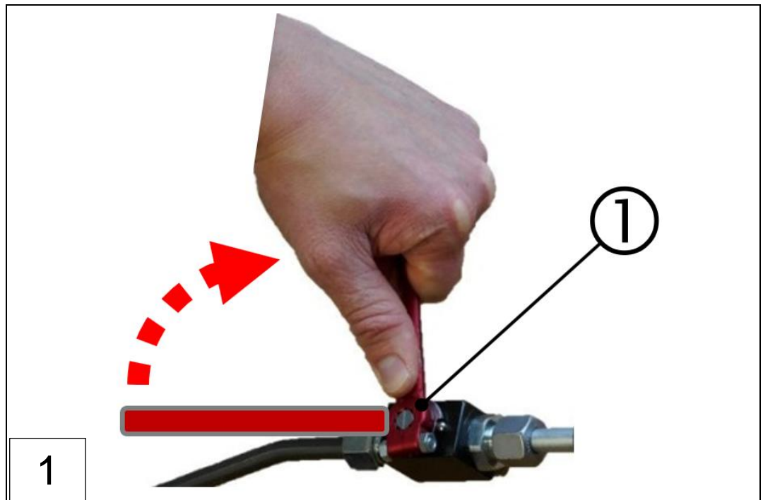
1: (关闭) 旋塞阀
