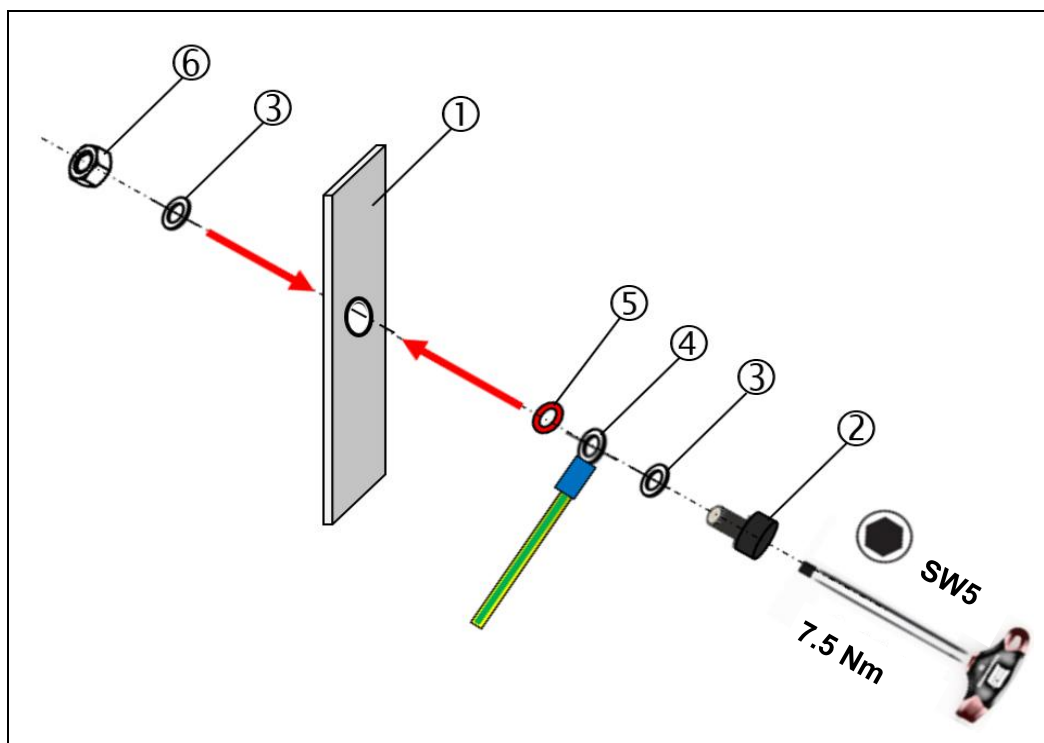
圖: 55： 接地连接的装配，VN200
