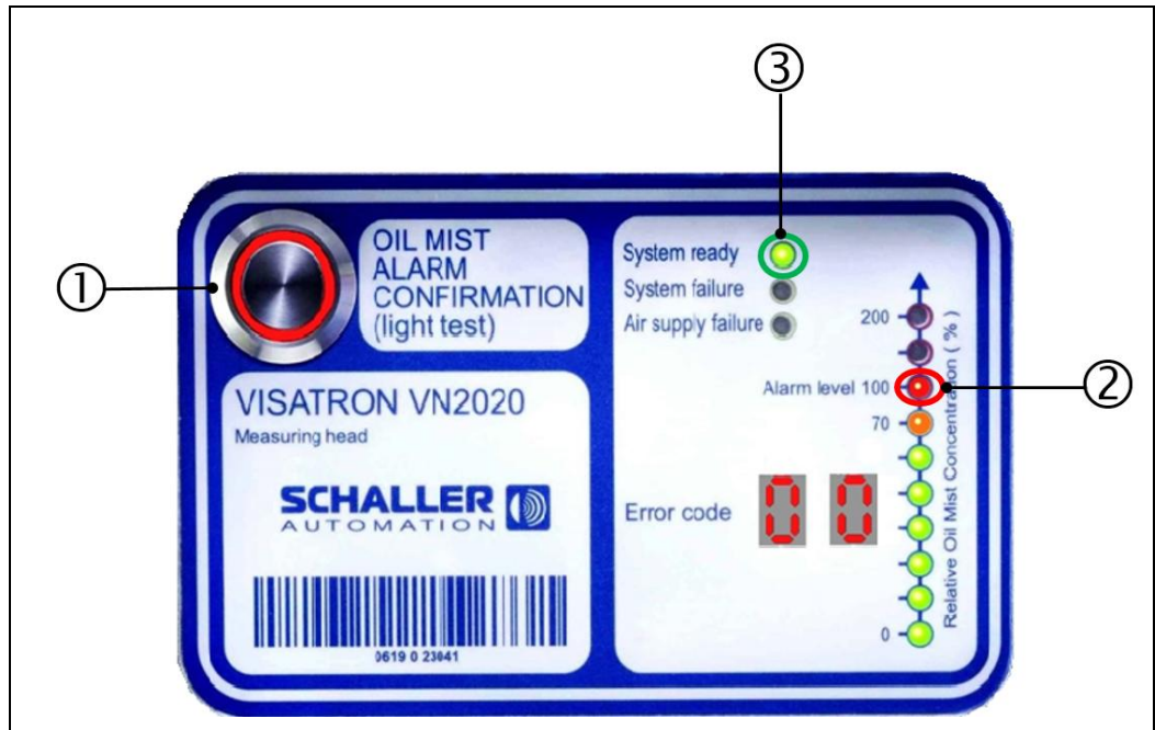
圖: 63: 功能测试, 首次投入使用, VN200 / VN200 EX
