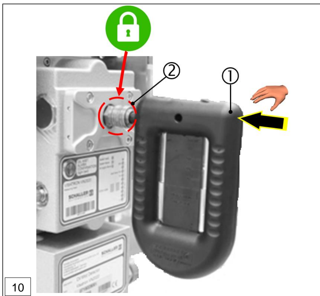
圖: 78: 更换空气滤清器滤芯, 压力控制器单元 (步骤 1 - 10)
