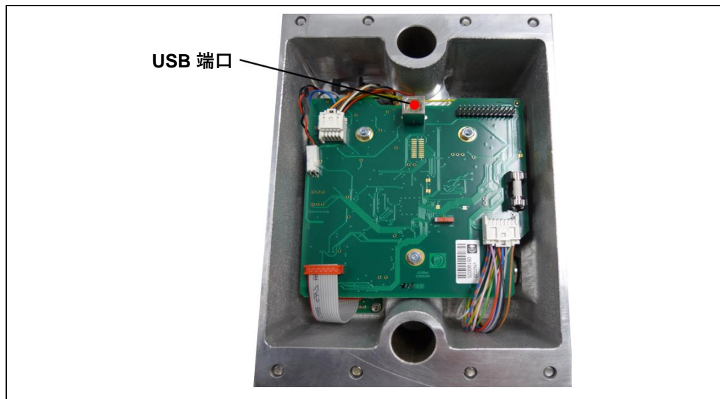
圖: 65: 测量附件 VN2020, 后视图, USB 端口
