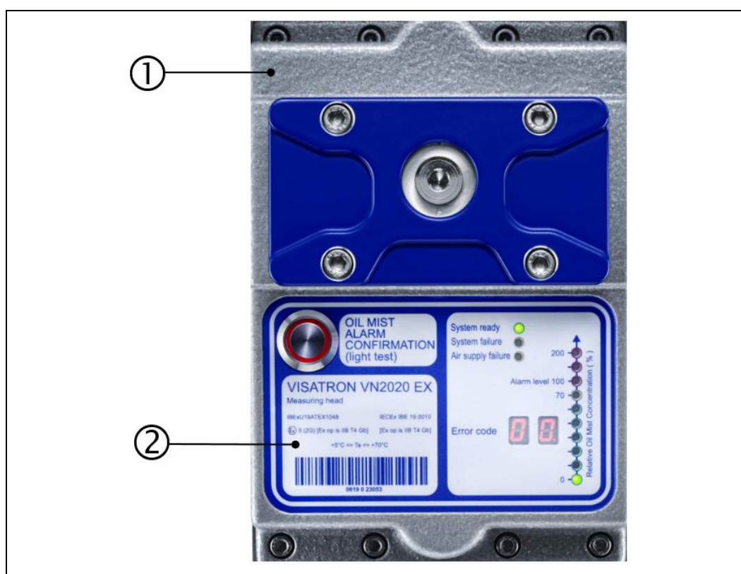
圖: 3: 铭牌, VISATRON® VN200 EX 测量附件
