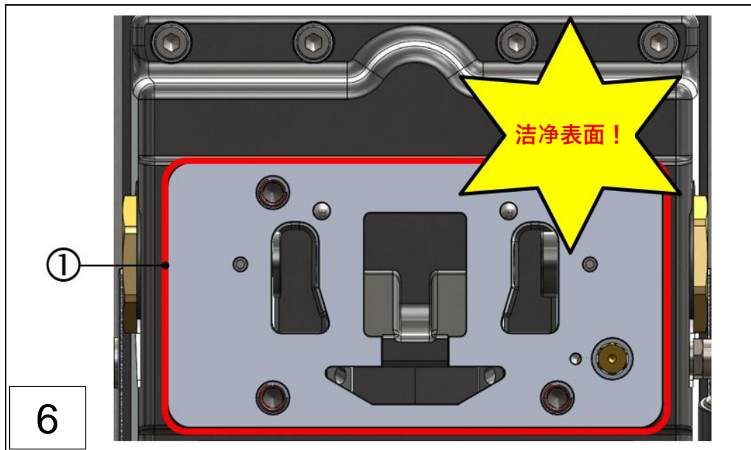
1: 密封面 (已清洁)、检查盖
