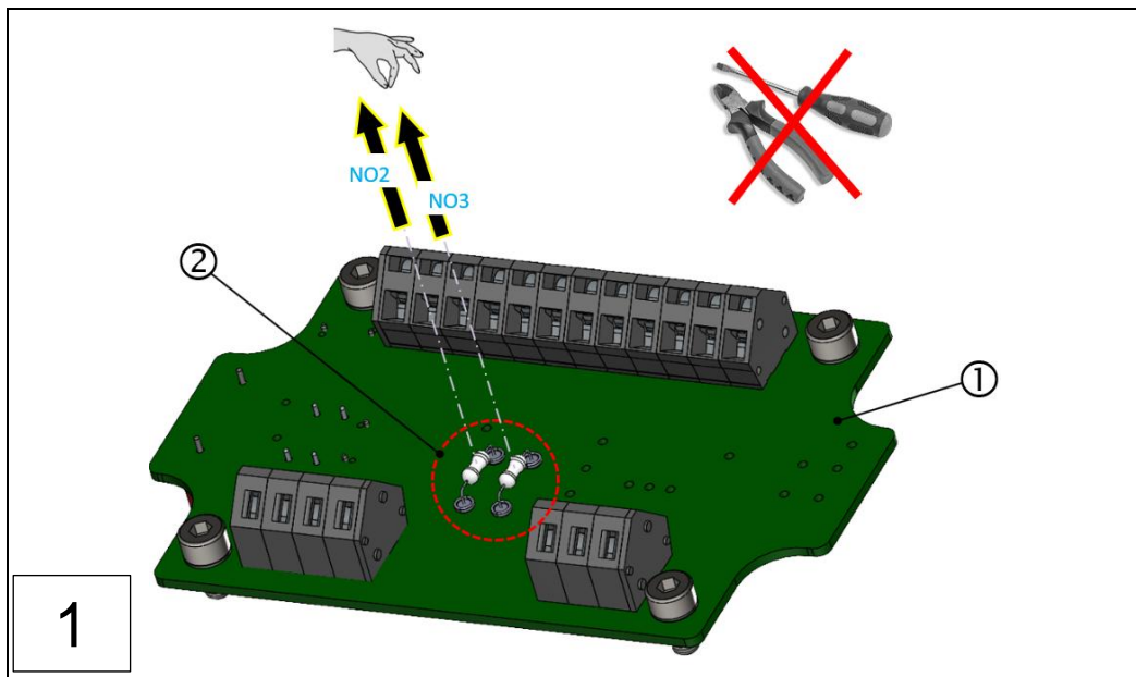
1: 接线电路板, VN2020 接线盒
