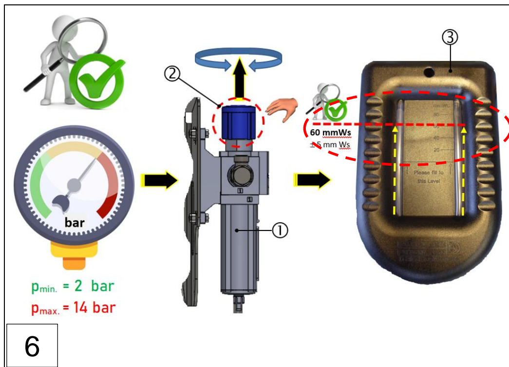
Abb.: 45 :Einstellen des Unterdrucks am Messaufsatz, VN2020 EX-H2 (Schritte 1-6)
