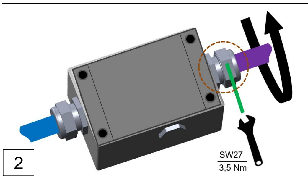
Abb.: 38 :Anschluss Remote Indicator II, Klemmenkasten, (Bsp.- Install., Montageschritte 1-2)
