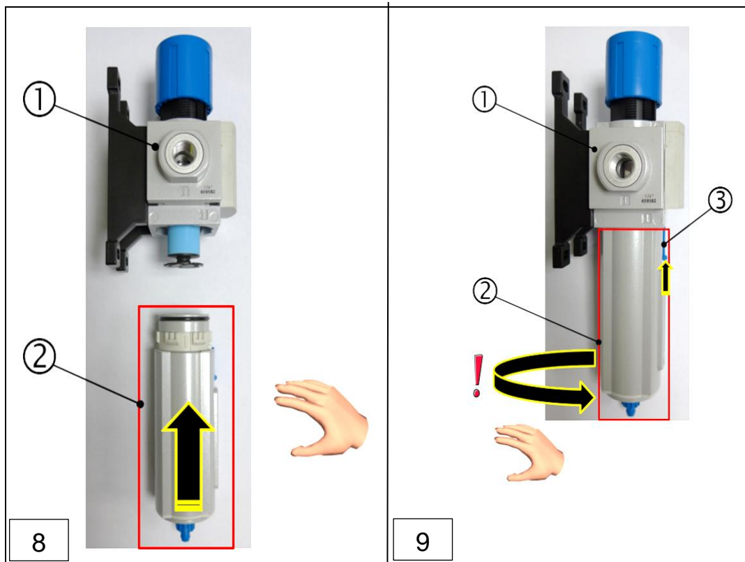
1: Druckregler- Einheit 2: Filterabdeckung 3: Verriegelungshebel
