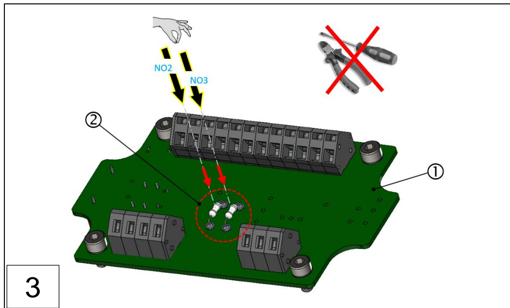
Abb.: 33 : Klemmenkasten VN2020 EX-H2: Drahtbruchwiderstände einsetzen (Schritte 1-3)
