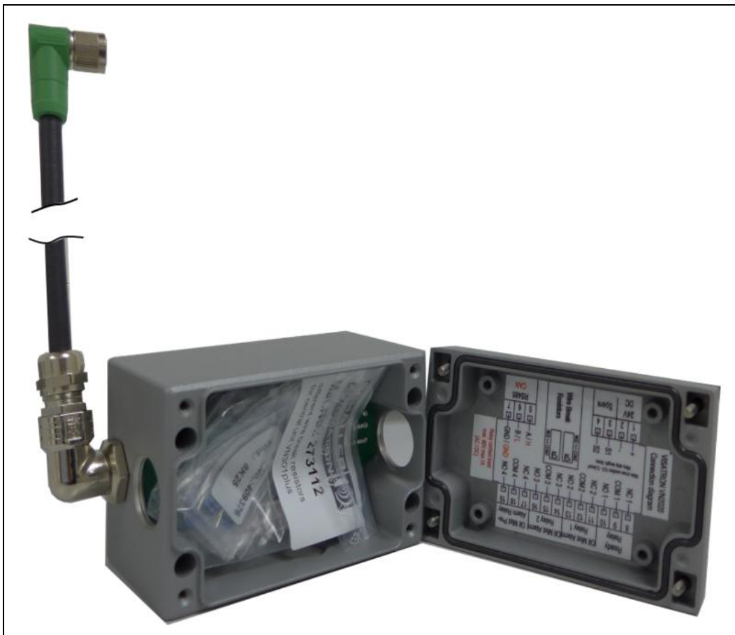
Abb.: 75 :Klemmenkasten (Ersatzteil), VN2020 EX-H2
