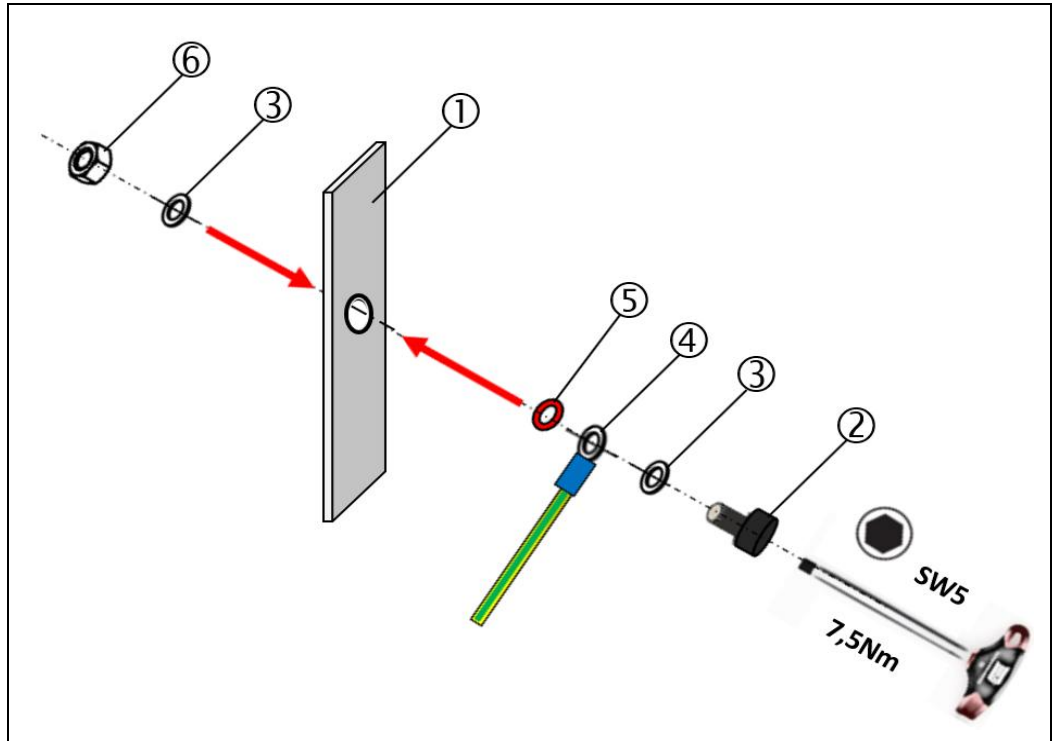
Abb.: 43 :Montage Erdungsanschluss, VN2020- Baureihe
