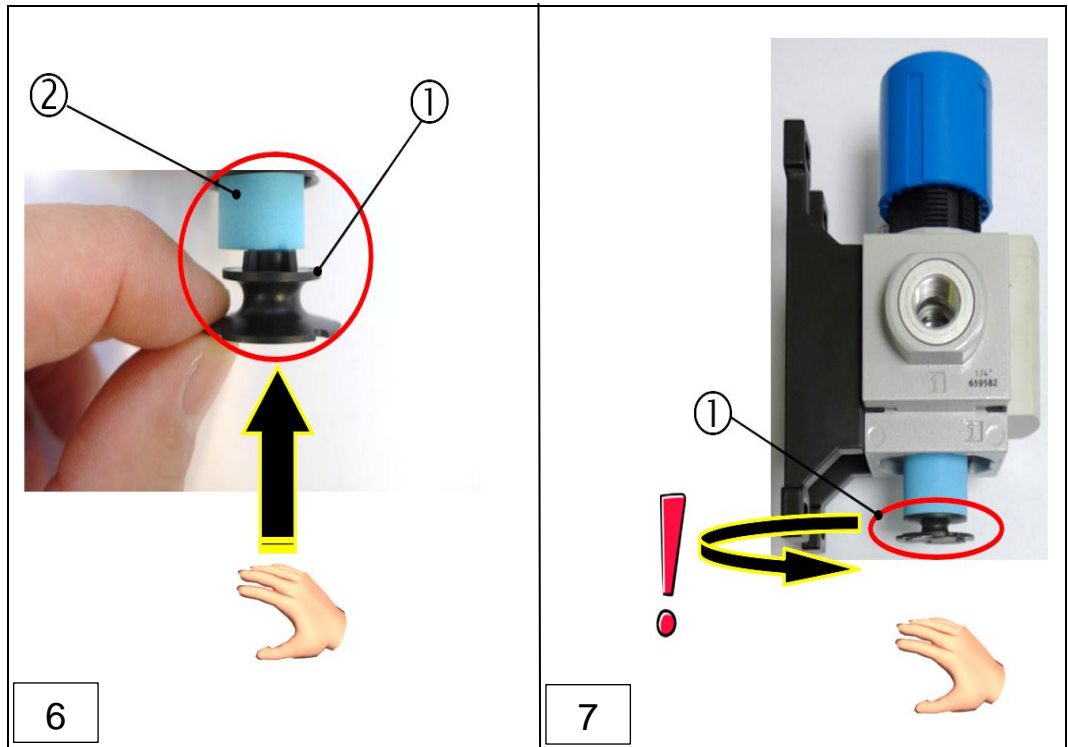
1: Kunststoff- Drehscheibe
