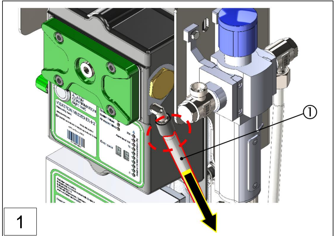
1: Druckluftleitung "Messaufsatz", VN200 EX-H2
