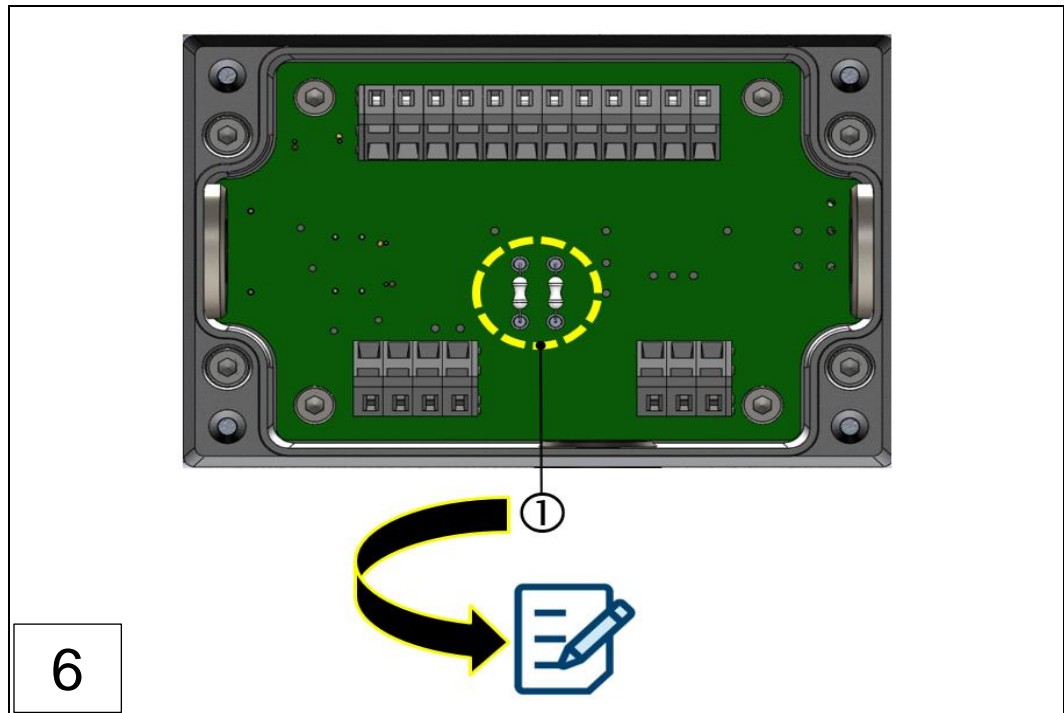
1: Drahtbruchwiderstände
