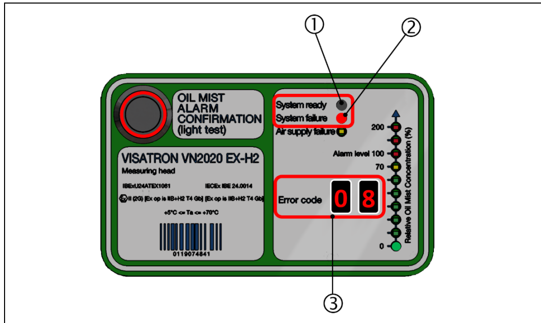
Abb.: 81 :Messaufsatz VN200 EX-H2: Status- Anzeige „System- oder Gerätefehler“
