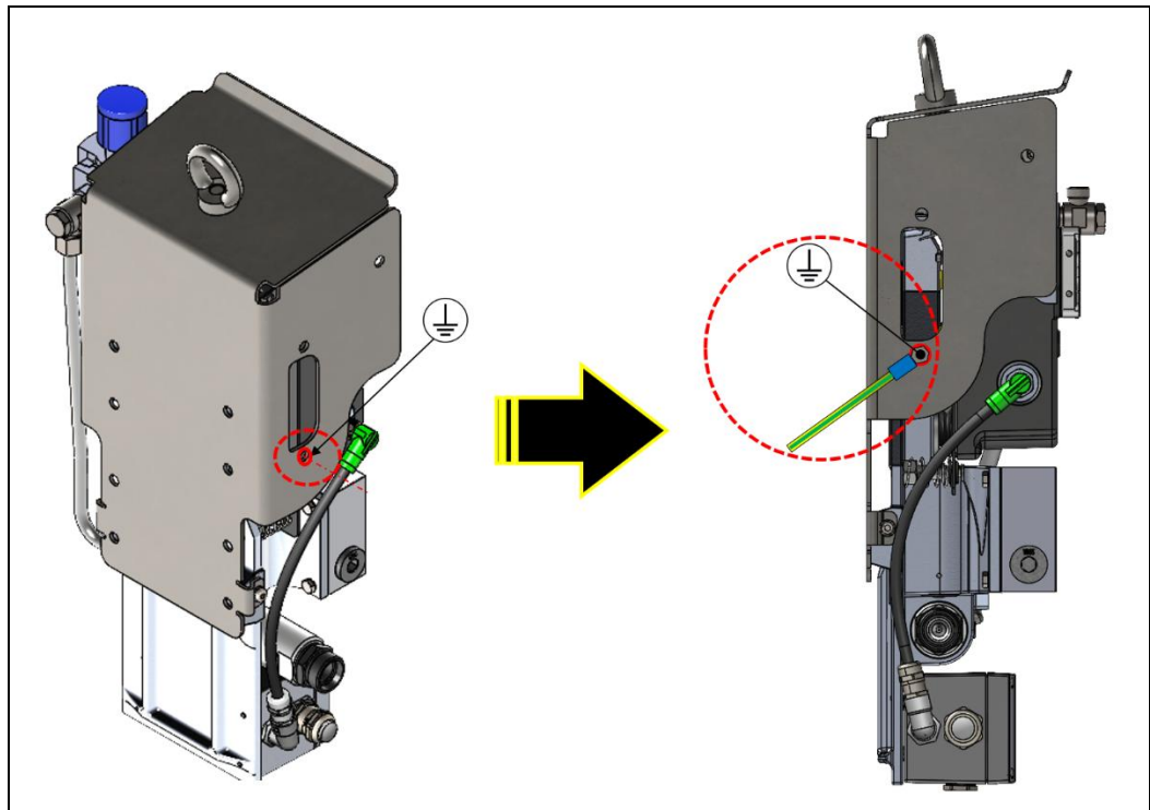
Abb.: 42 :Position und Installation, Erdungsanschluss, Schutzhaube VN2020- Baureihe
