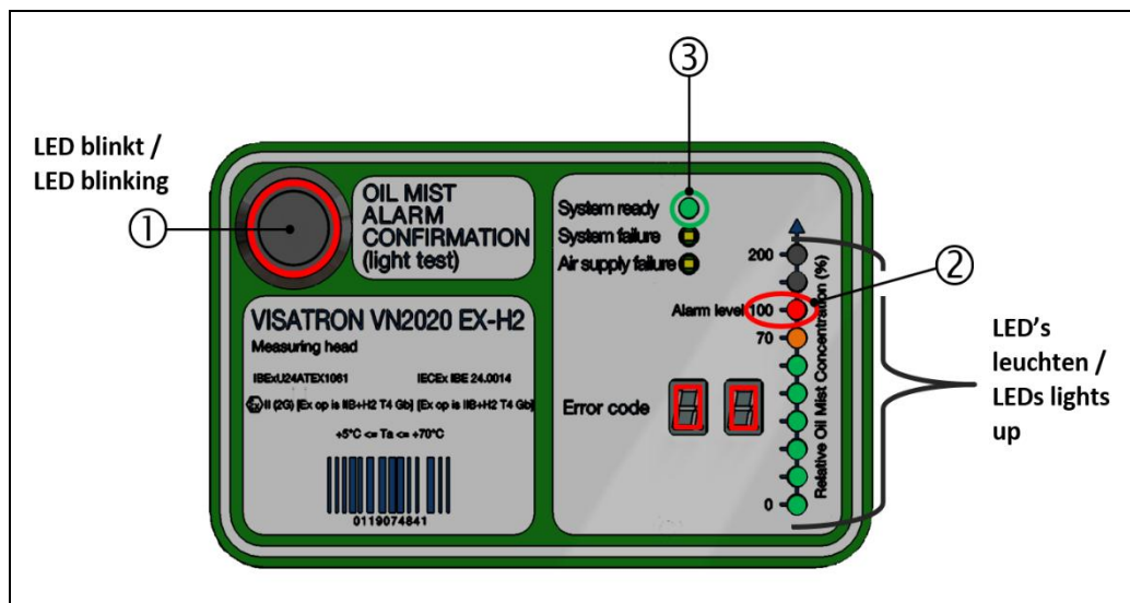
Abb.: 59 :Messaufsatz VN2020 EX-H2: Status- Anzeige „Alarm“ bei 100% ÖNK
