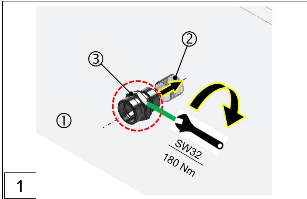
1: Motorwand 2: Anschlussgewinde, Motorwand 3: Gerader Einschraubstutzen L22
