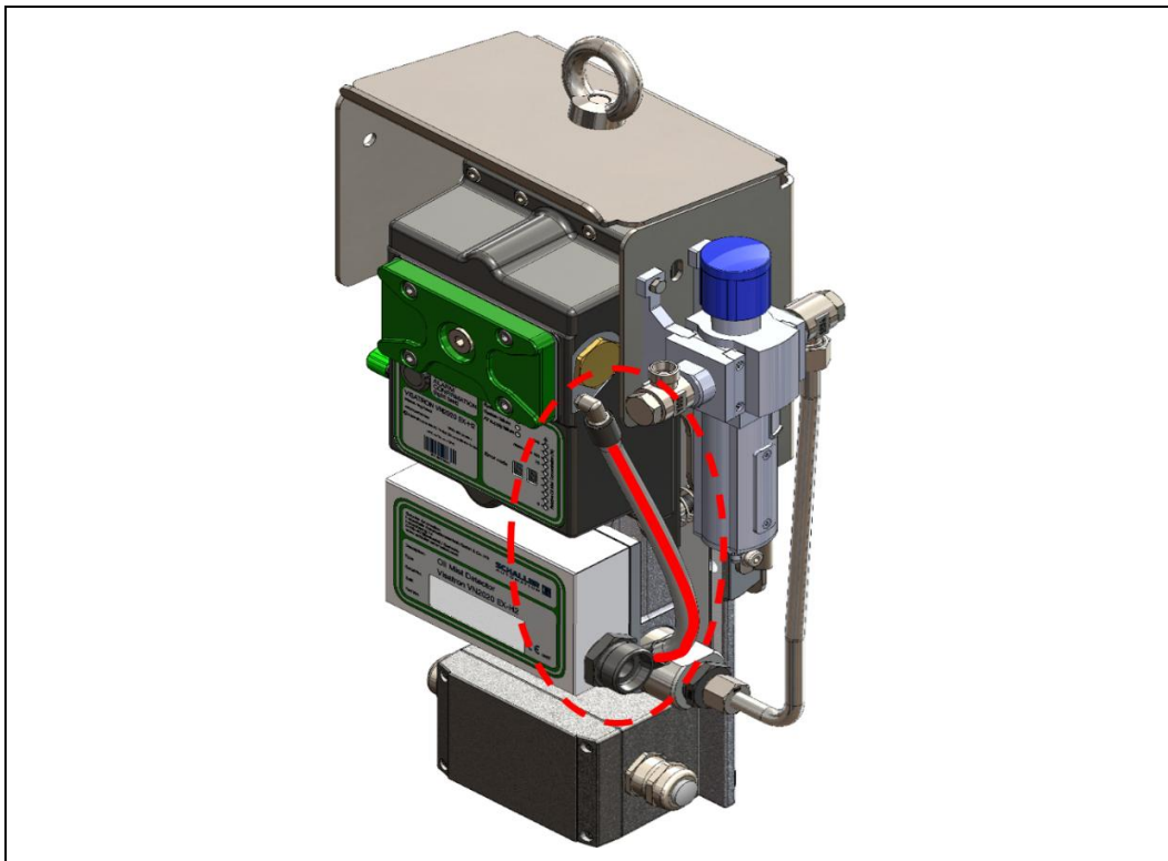
Abb.: 79 :Verbindungsleitung, Ölnebeldetektor VN2020 EX-H2
