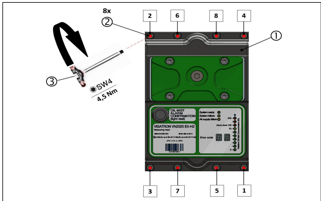
Abb.: 55 :Montage Messaufsatz VN2020 EX-H2
