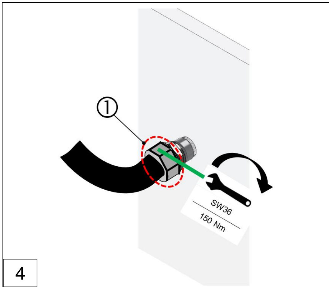
Abb.: 25 :Montage der Rückführleitung, VN2020 EX-H2 (Schritte 1-4)
