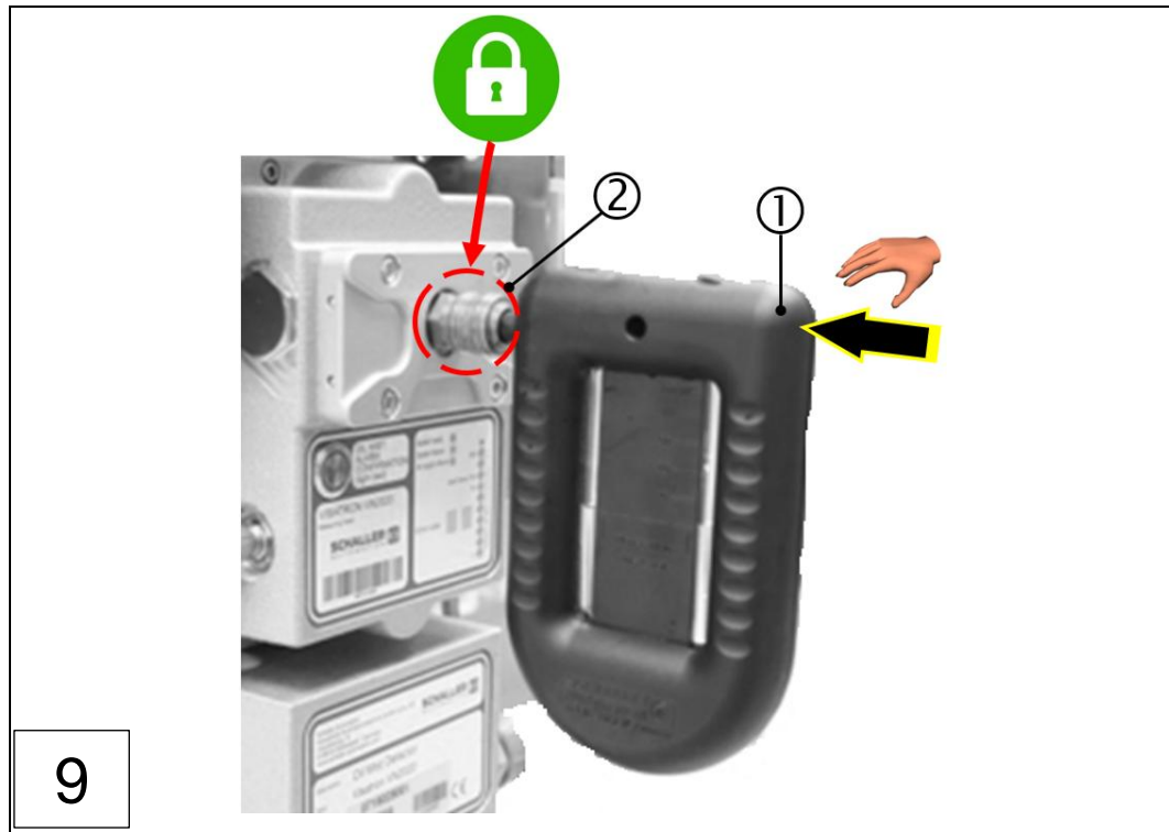
Abb.: 71 :Messaufsatz VN2020 EX-H2 austauschen, (Schritte 1 - 9)
