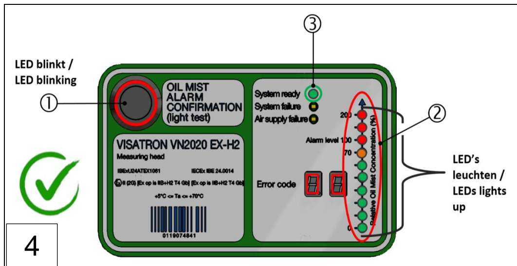
Abb.: 67 : Funktionstest mit Testnebel (Schritte 1-4)
