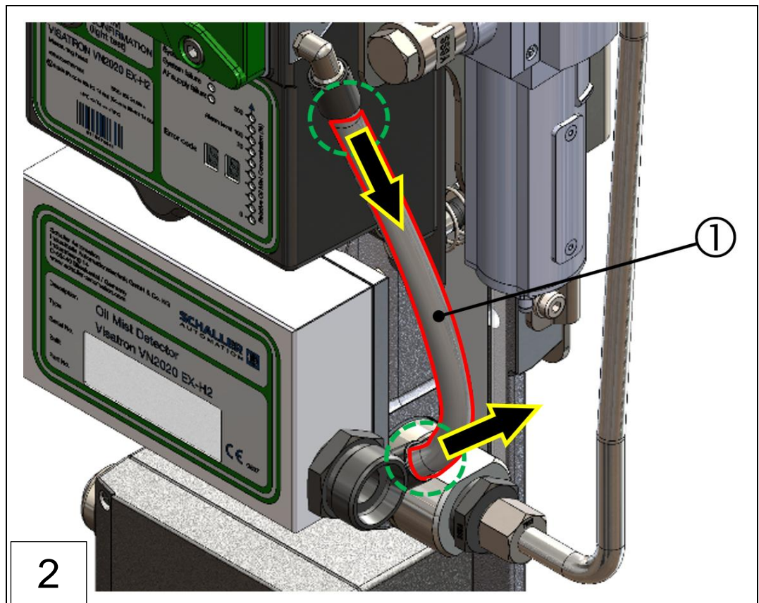
1: Verbindungsleitung (alt)
