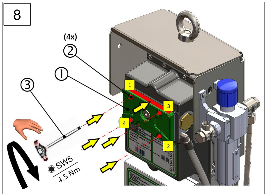
Abb.: 62 :Reinigung der Lichtstrecke VN2020 EX-H2 (Schritte 1- 8)
