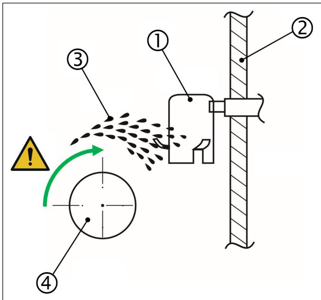
Abb.: 19 :Montageempfehlung der Motorwandverschraubung (Ansicht vom Kurbelwellenende)
