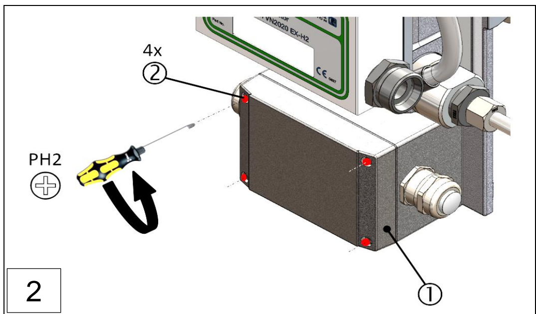
1: Deckel „Klemmenkasten“
