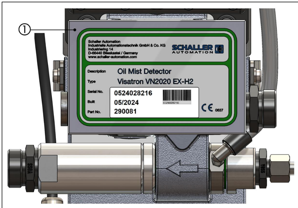
Abb.: 68 :Anschlusskasten, Ölnebeldetektor VN2020 EX-H2
