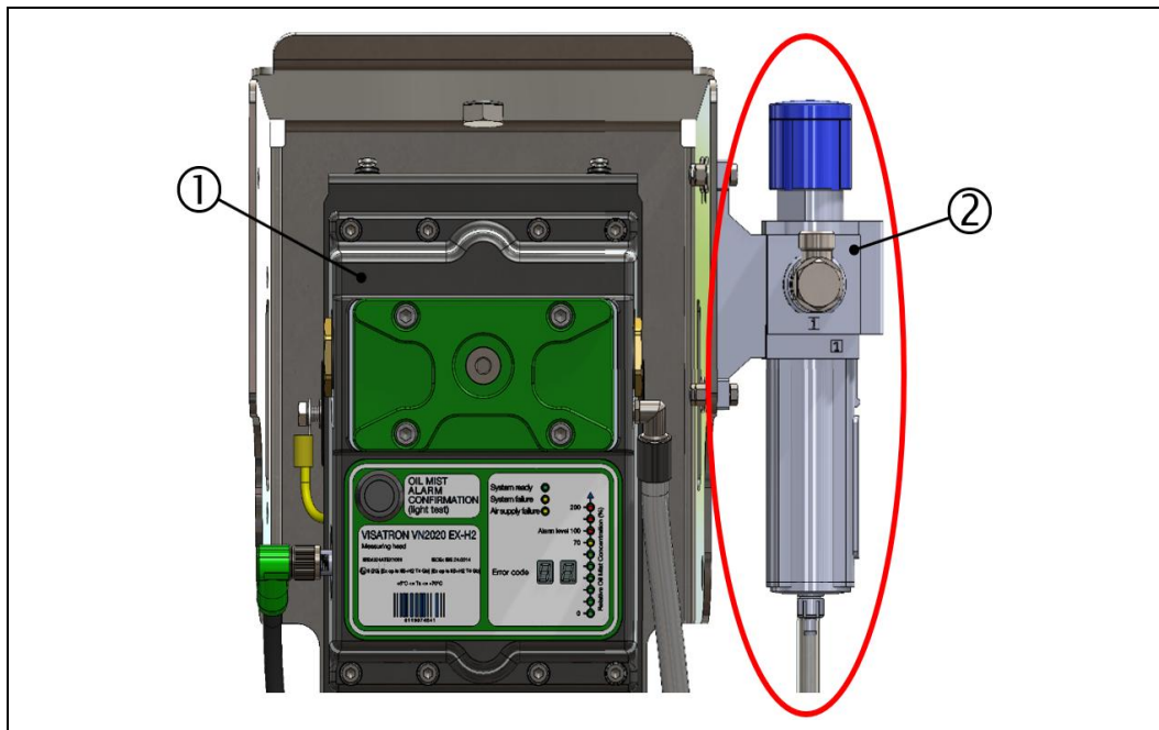
Abb.: 63 :Druckregler- Einheit, Ölnebeldetektor VN2020 EX-H2
