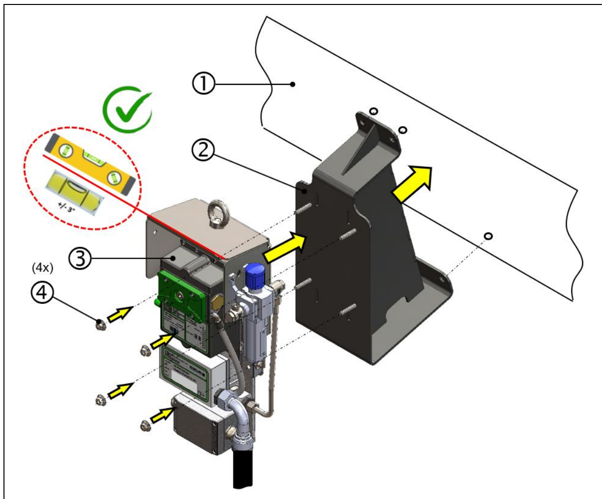
Abb.: 15 :Montagevorgang, VN2020 EX-H2 mit Konsole und Schutzhaube
