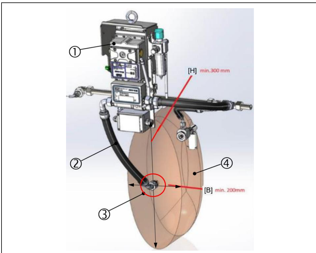
Abb.: 24 :Position Rückführungsrohr, VN2020 EX-H2
