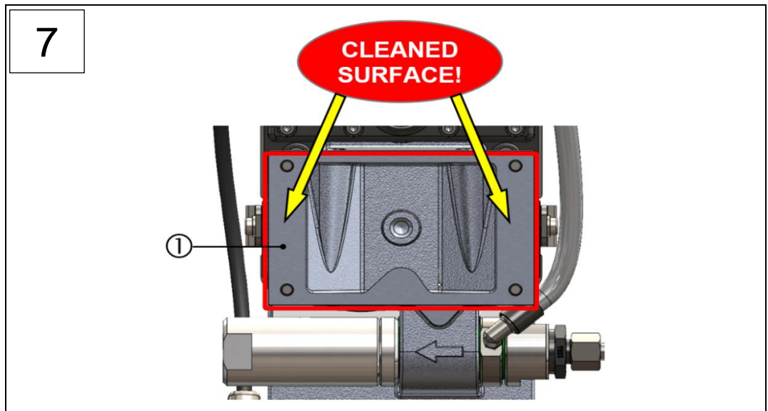
1: Dichtungfläche "Anschlusskasten"
