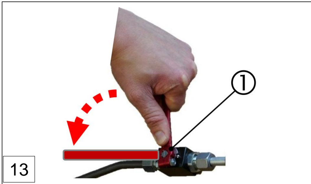
Abb.: 69 :Austausch Dichtung am Anschlusskasten (Schritte 1- 13), VN2020 EX-H2
