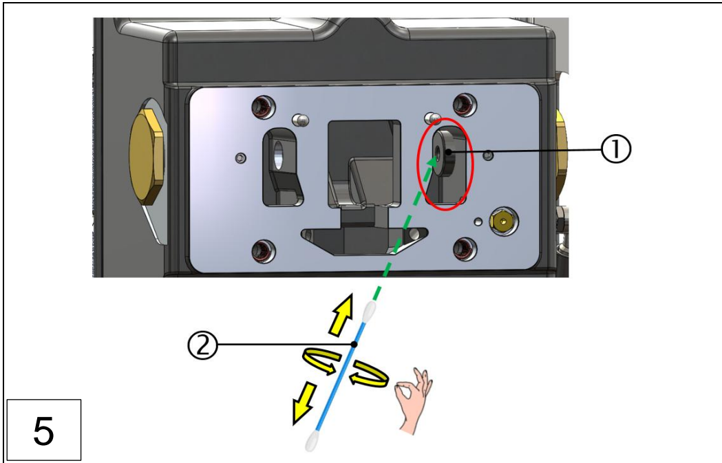
1: Diodenglas, rechts
