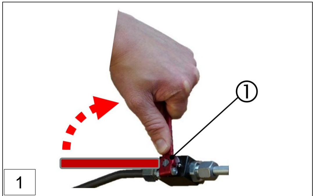
1: Absperrhahn (schließen)
