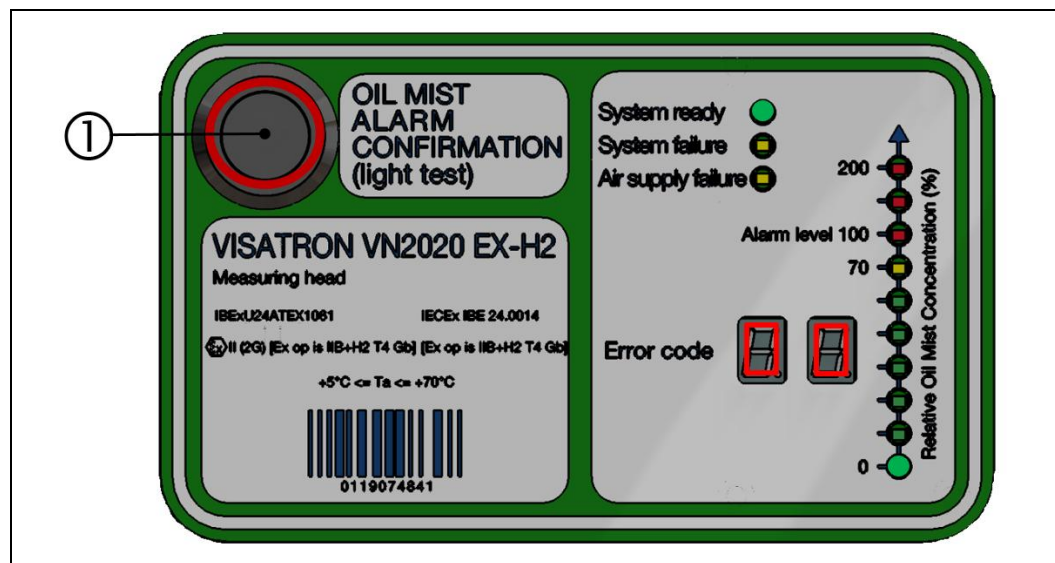
Abb.: 57 :Messaufsatz VN2020 EX-H2: LED- Check (Leuchtentest)
