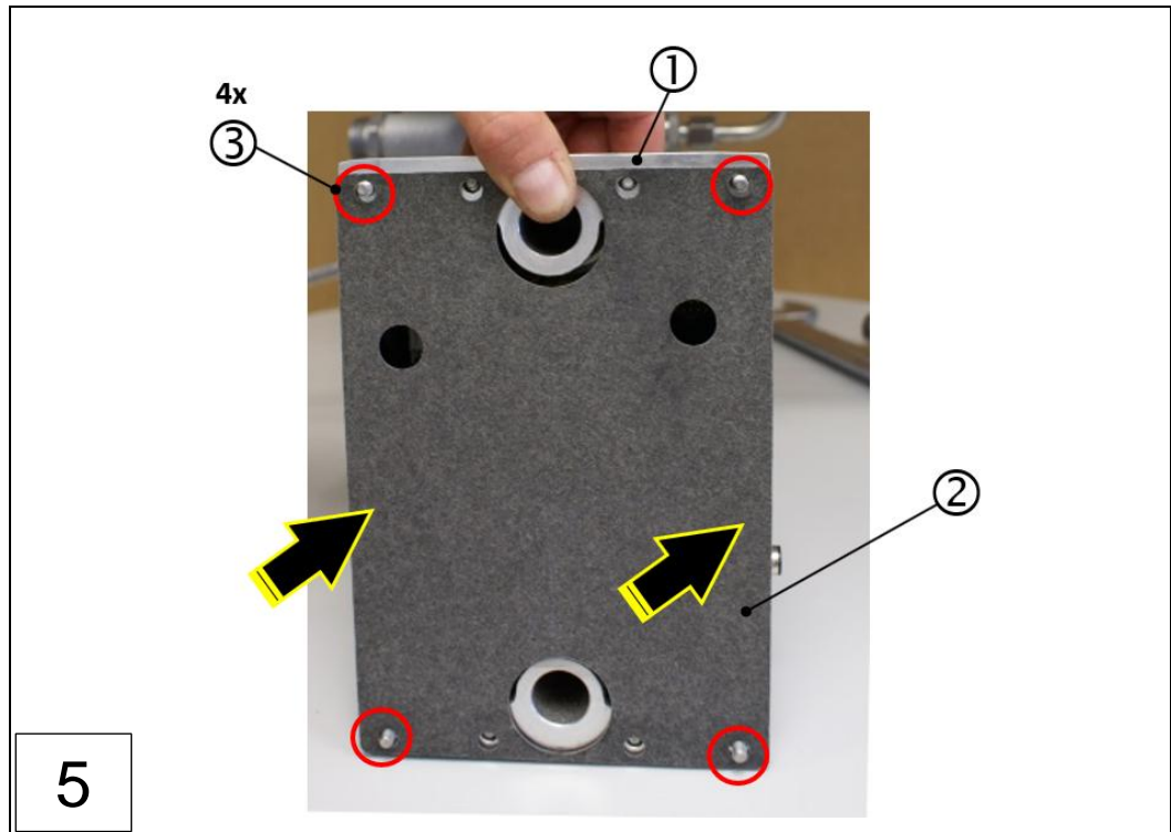
1: Messaufsatz (Neu), VN2020 EX-H2 2: Dichtung (Neu) "Messaufsatz" 3: Halsschrauben
