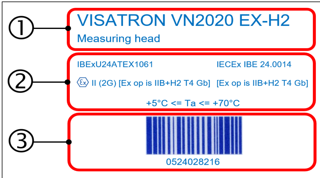
Abb.: 2 : Typenschild, Messaufsatz VISATRON ® VN2020 EX-H2
