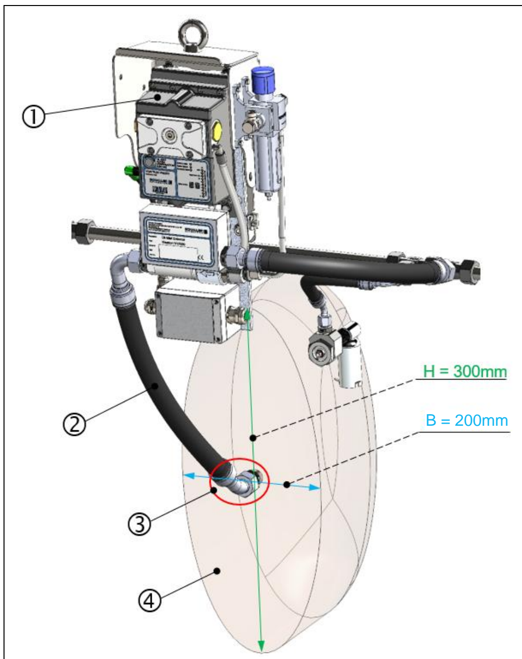
Fig. : 10 : Position de la conduite de retour, KIT de mise à niveau VN2020
